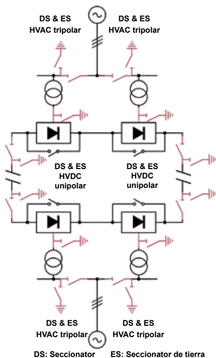
DS: Seccionador ES: Seccionador de tierra
